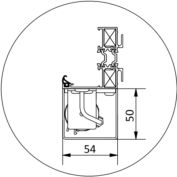
Détail - C Ech : 1/3
